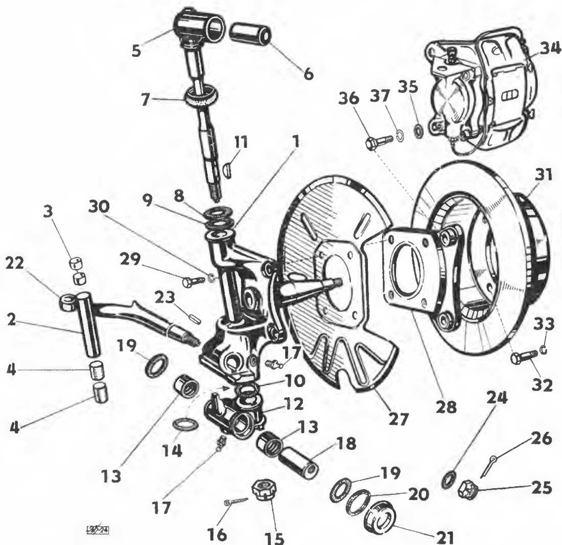
Čepy kol s brzdovým ústrojím — Wheel Pivots with Brake Mechanism Pivots de roues avec mécanisme de frein — Achsschenkel mit Bremsvorrichtung
