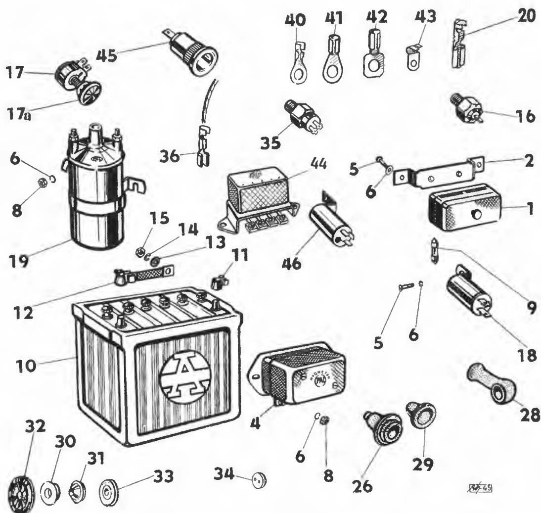
Elektrické příslušenství — Electrical Accessories Accessoires électriques — Elektrisches Zubehör
