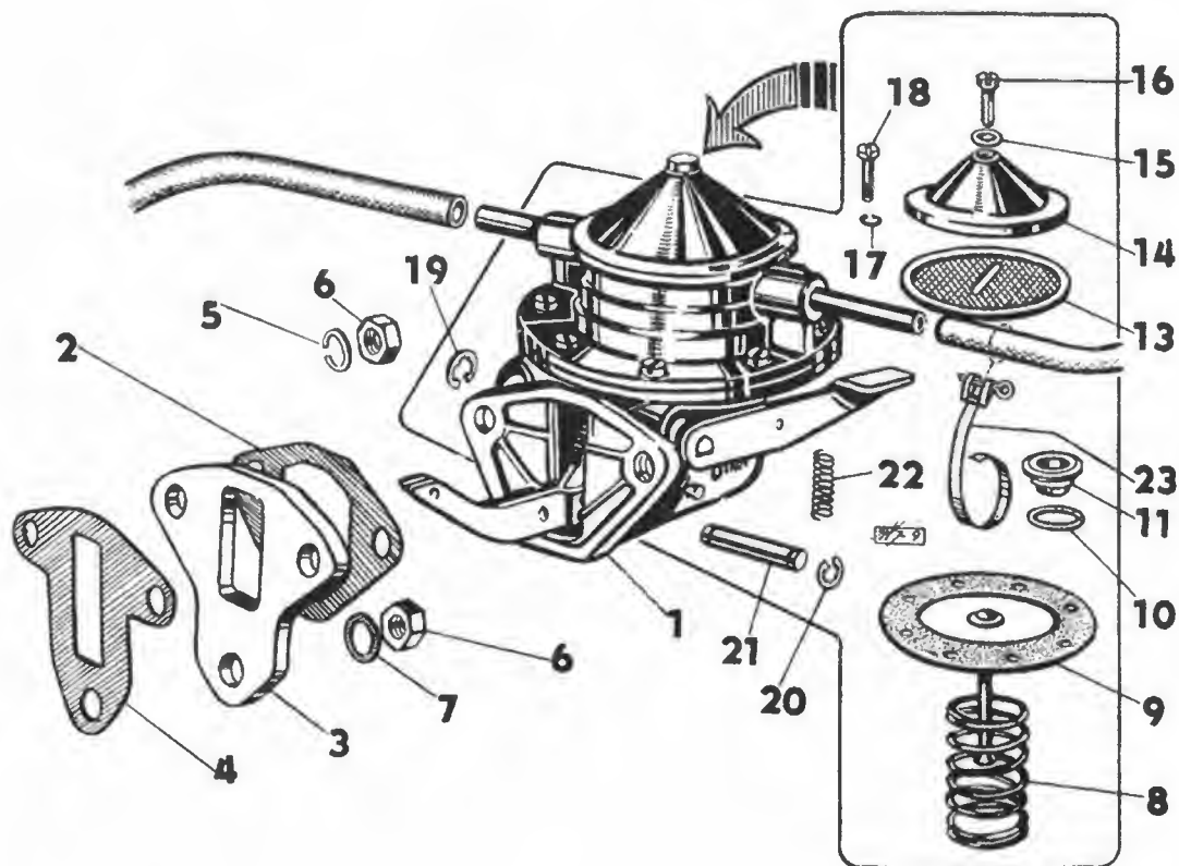
Palivové čerpadlo — Fuel Pump — Pompe à essence — Kraftstoffpumpe
