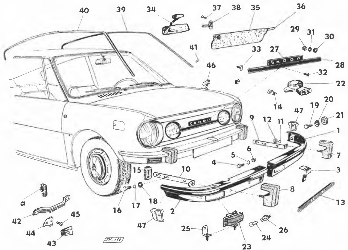
Přední nárazník a ozdobné lišty — Front Bumper and Decorative Mouldings Pare-choc avant et moulures décoratives — Vordere Stosstange und Zierleisten
