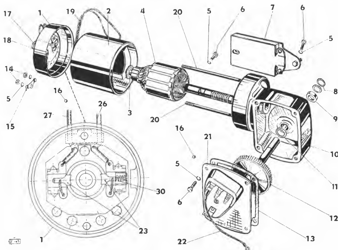
Náhradní díly stírače – Spare Parts of Windscreen Wiper Pièces de rechange d'essuie-glace – Ersatzteile des Scheibenwischers
