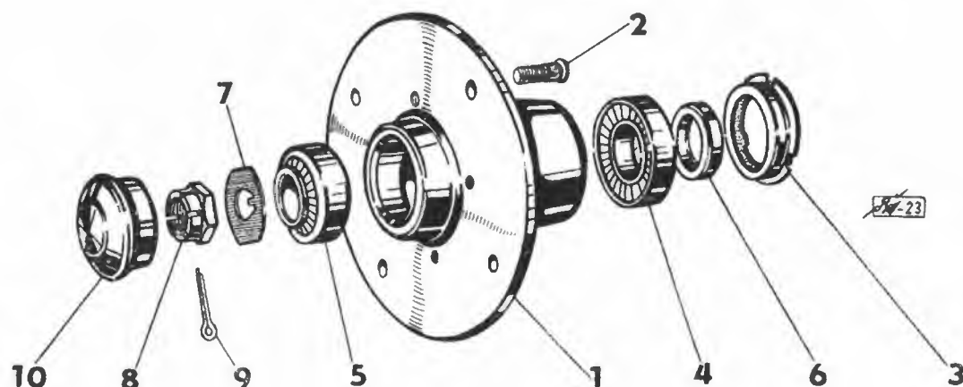
Hlava kola s uložením — Wheel Head with Bearings Tête de roue avec logement — Radnabe mit Lagerung
